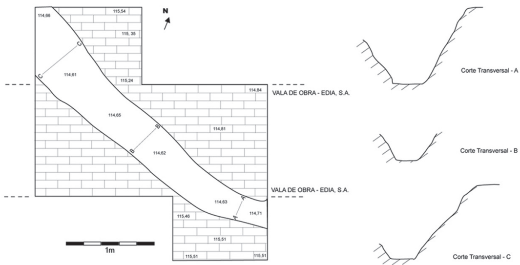
Figura 3 – Planta e secções transversais de segmento de “fosso” identificado em Barranco do Rio Seco 4.
